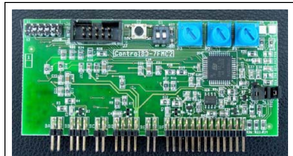
STEVAL-IHM002V1
